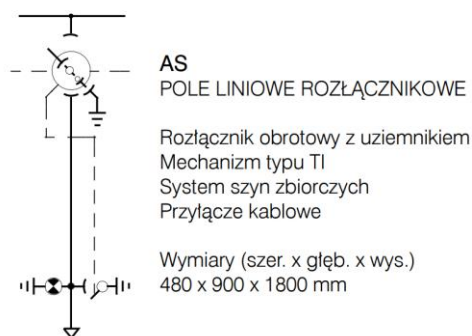
Rysunek nr 8: Schemat pola liniowego AS.
